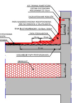
SZCZEGÓŁ 5 OBRÓBKA KOMINA/ŚCIANY
